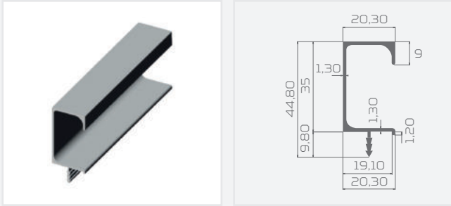
KOD: 60335 SÜPÜRGELİK DÜZ (FOLYOLU)
