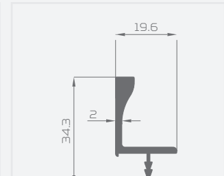
KOD: 60711 GOLA FİTİLSİZ ÜST PROFİLİ (FOLYOLU)
