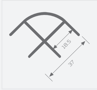
KOD: 60310 KÖŞE DÖNÜŞ (18'LİK)
