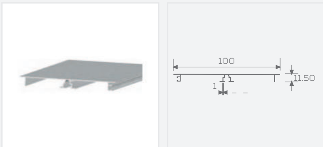
KOD: 60100 DÜZ BAZA (12'LİK) (FOLYOLU)
