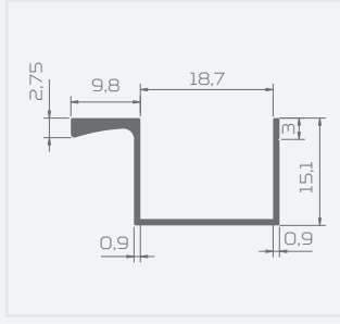
KOD: 60606 BOY KULP (FOLYOLU)
