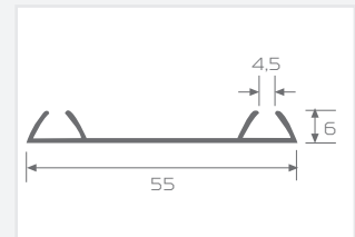
60270 / Alt Ray
