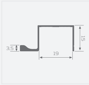
KOD: 60622 BOY KULP (FOLYOLU)
