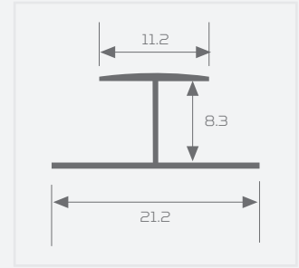
KOD: 60290 ÜST RAY (FOLYOLU)
