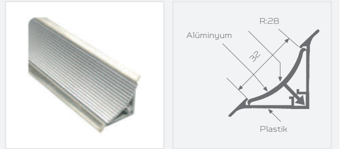
KOD: 60095 ÇİZGİLİ BAZA (10'LUK) (FOLYOLU)
