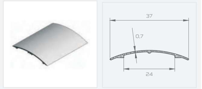
KOD: 60575 MERDİVEN BİTİM PROFİLİ
