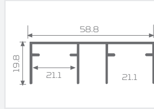
60025 / Üst Ray
