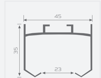
KOD: 60290 ÜST RAY (FOLYOLU)
