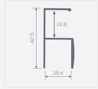
KOD: 60712 BOY KULP (FOLYOLU)
