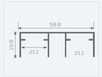
KOD: 60025 ÜST RAY (FOLYOLU)
