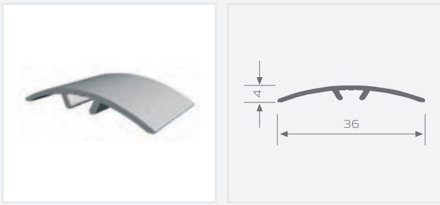
KOD: 60570 MERDİVEN BİTİM PROFİLİ
