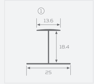
KOD: 60405 H PROFİL (8'LİK)
