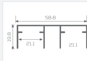
60025 / Üst Ray
