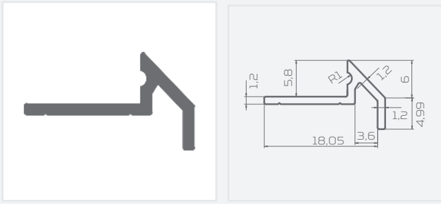
KOD: 60200 EŞİK ÇİTASI GENİŞ BANTSIZ
