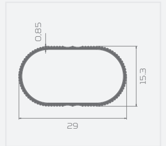
KOD: 60171 OVAL ASKI BORUSU
