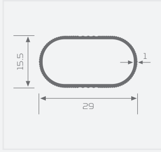
KOD: 60160-60165 DAİRE ASKI BORUSU
