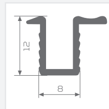
60014 / Alt Ray
